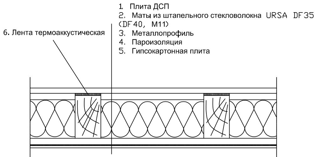
Решение пола над отопляемыми помещениями
